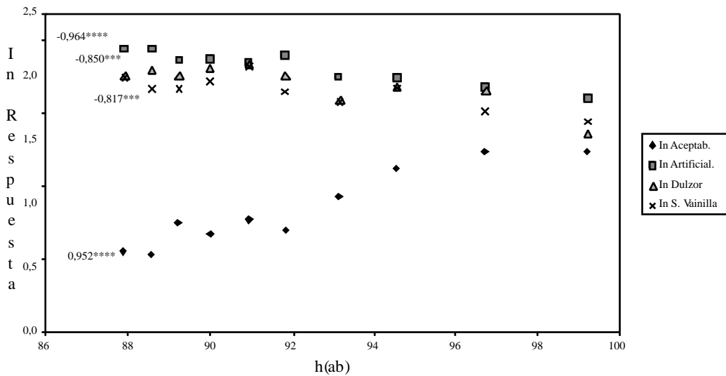
Figura 4. Diagrama de dispersión - In Respuesta en función de la cantidad de tono - y correlación
