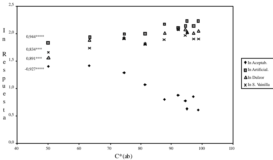
Figura 3. Diagrama de dispersión - In Respuesta en función de la cantidad de color (croma) - y correlación
