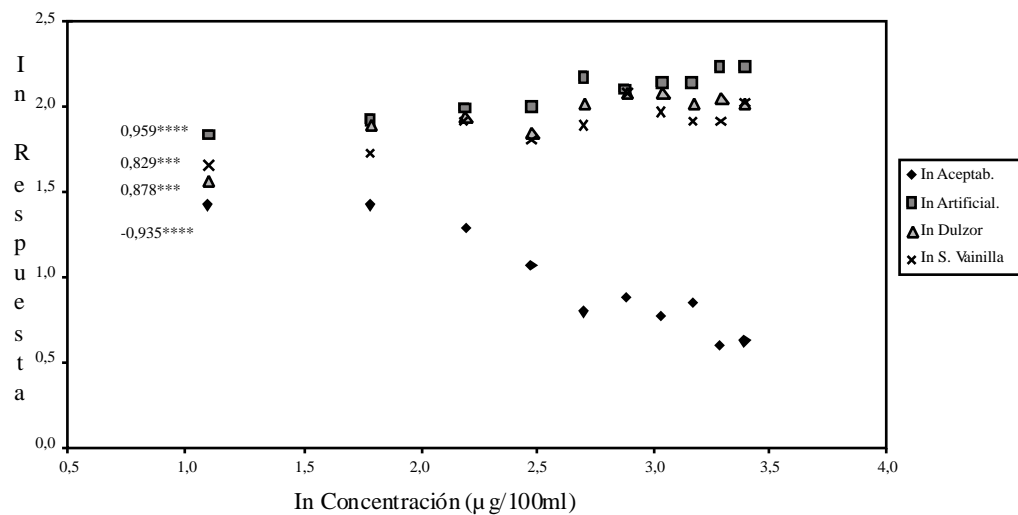
Figura 1. Diagrama de dispersión - In Respuesta en función de In concentración de tartracina - y correlación
