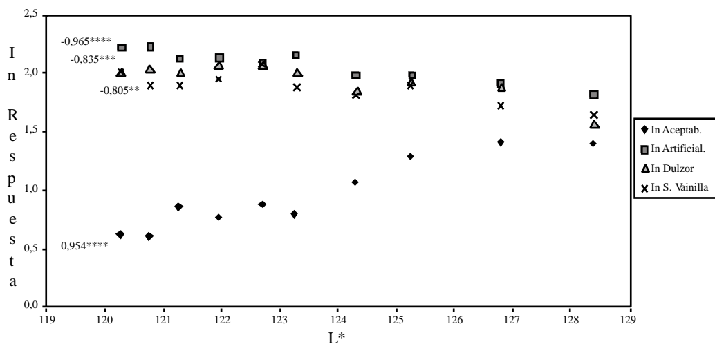
Figura 2. Diagrama de dispersión - In Respuesta en función de la claridad - y correlación
